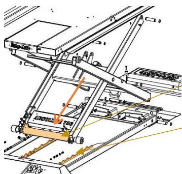
Figura 3 – Sistema di arresto meccanico
