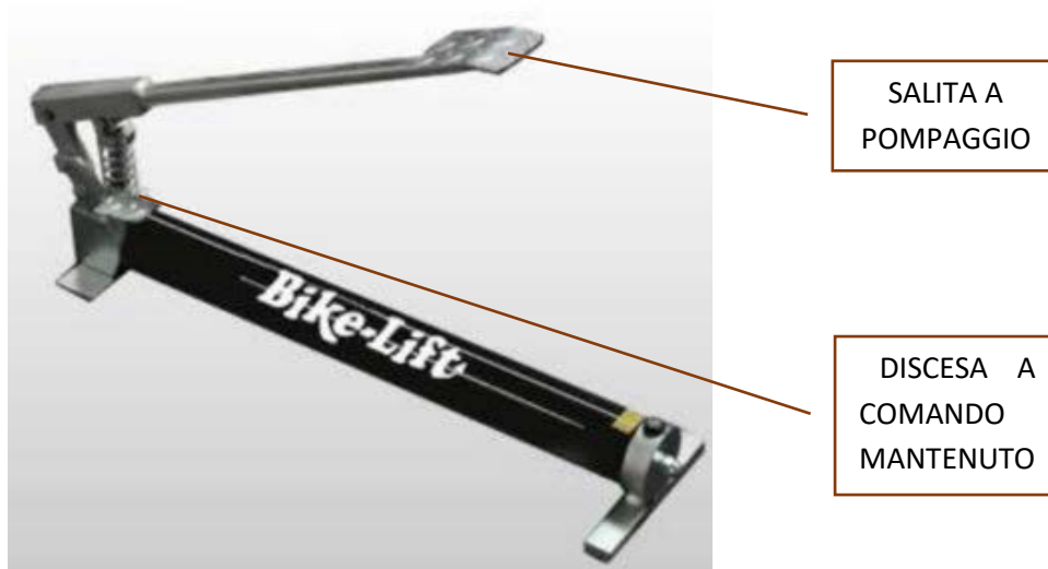
Figura 7 – Pompa idraulica a pedale
