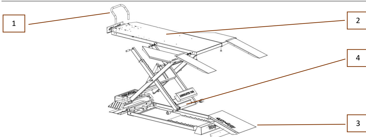
Figura 6 –modello generale di sollevatore
